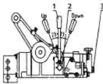
Рис.2. Гидравлический подъемник.
