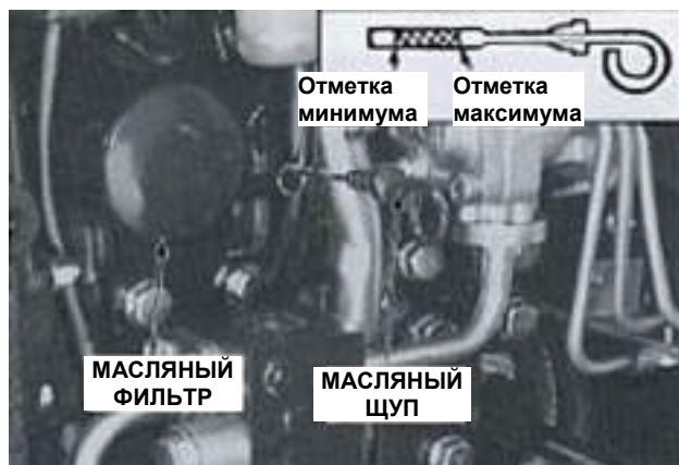
Рис. 49. Масляный щуп и фильтр
