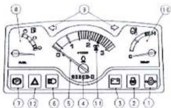
Панель инструментов
