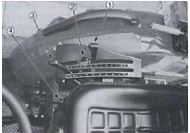
Рис. 35. Двухрычажная система управления гидроподъемником
