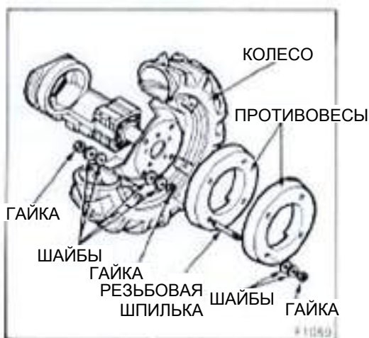
Рис. 45. Колесные противовесы
