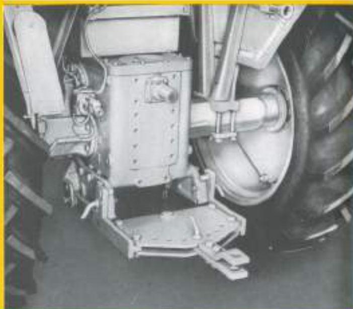
Attelage « Trainé ».
