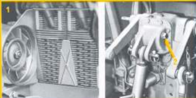
1. Refroidissement. 2. Niveau remplissage du relevage hydraulique.
