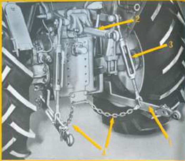
Attelage « 3 points » (rotant).
