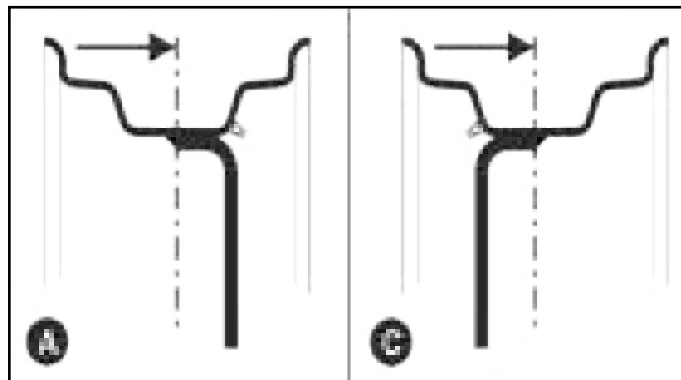
Impostazioni carreggiata / ruote a trazione anteriore meccanica (MFWD). MFWD con Cerchi Saldati in 2 posizioni / Versione V Tread Settings / MFWD FRONT wheels. MFWD with 2 Positions welded Rim / V Version
